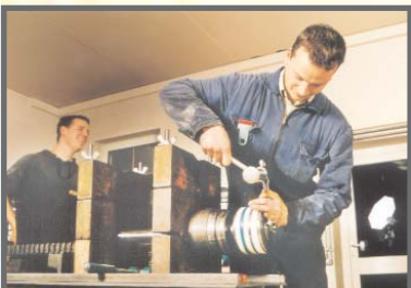
Montage der neuen Dichtelemente
