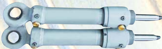
2 Hydraulikzylinder nach dem Zusammenbau und der Druck/Dichtheitsprüfung
